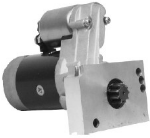
18492 12V/9T/1.4KW
